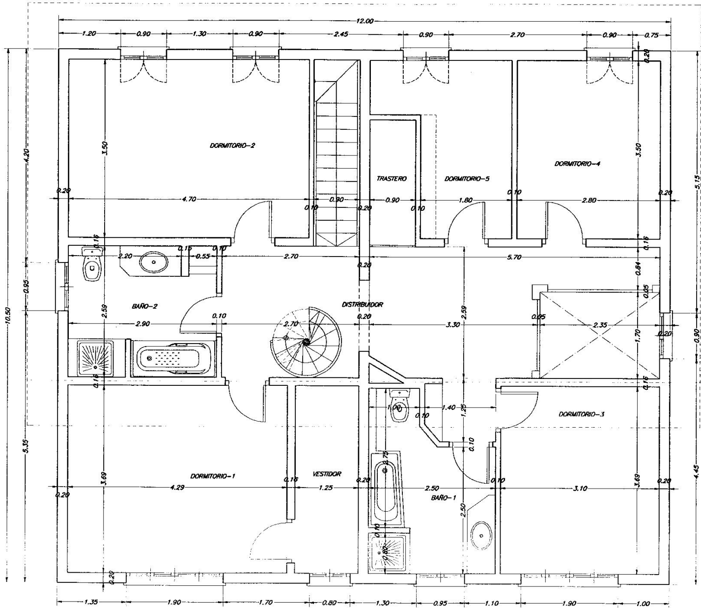
PLANTA PISO
